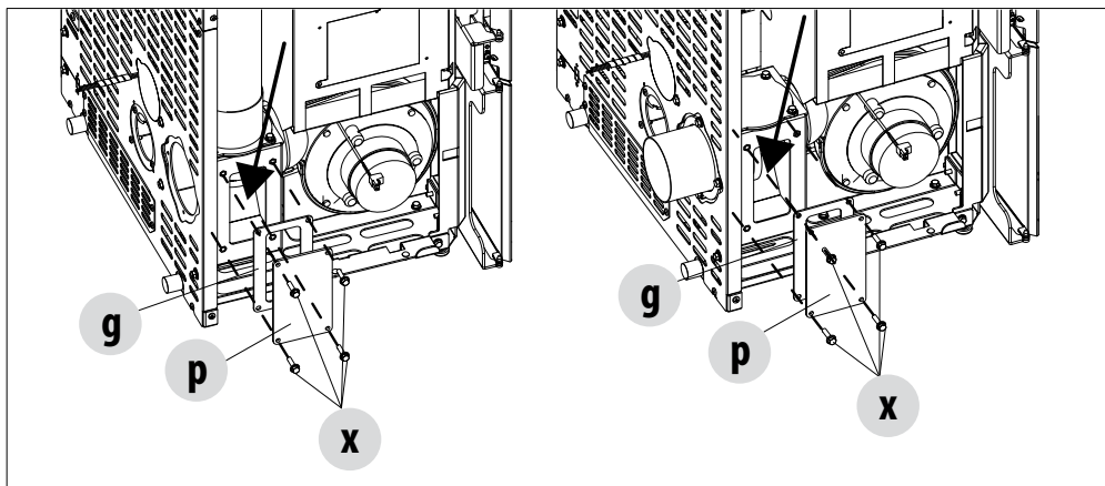
NETTOYAGE DE LA SORTIE DE FUMÉES SUPÉRIEURE
